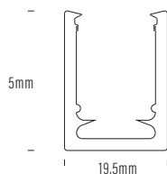
AQS-500-ACC-AL-04 1m Polycarbonate
