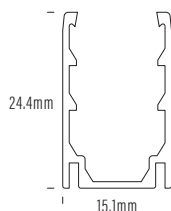
AQS-420-ACC-01 1m Aluminium
