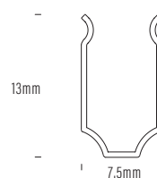
AQS-402-ACC-03 Aluminium Clip
