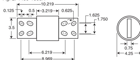
Fig. 2: 1400-1600A
