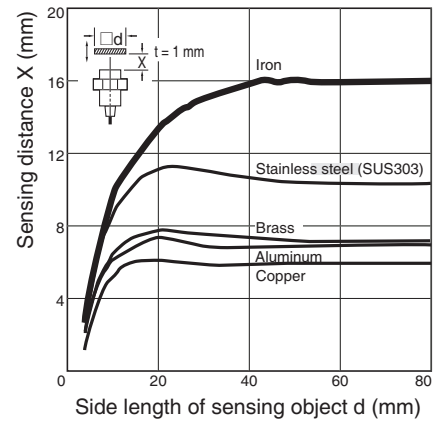
E2A-M18□N16/E2A-S18□N16
