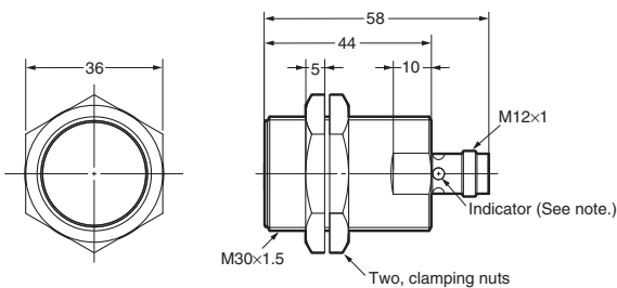
E2A-M30KS15-M1-□□/E2A-S30KS15-M1-□
