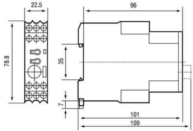
RZ7-FS (2 C/O)
