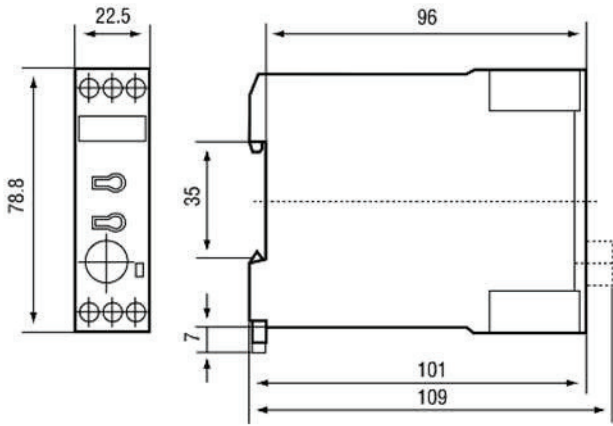
RZ7-FS (1 C/O)
