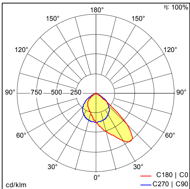
TE_LEO_FLEX_80W_840_FLEX1.ldt
